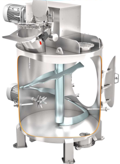
縦型1軸混合機
